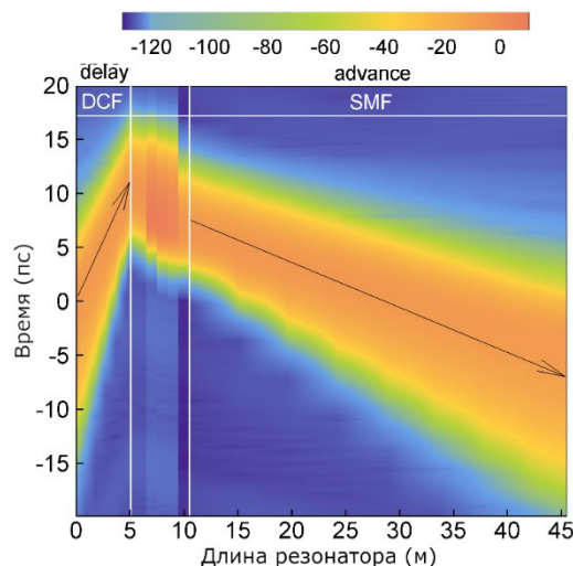
Рис. 1. Эволюция импульса на одном обходе резонатора.
