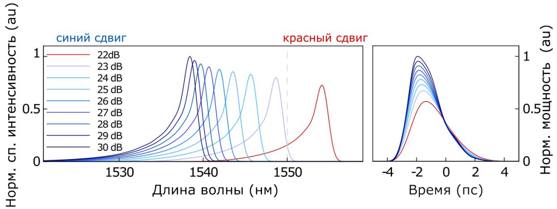
Рис. 2. Спектральные (слева) и временные (справа) профили в зависимости от коэффициента усиления малого сигнала (тока инжекции) при кумулятивной дисперсии \beta_2^{\text{cum}} = -0.18 \text{ ps}^2 и ширине спектрального фильтра 40 нм.
